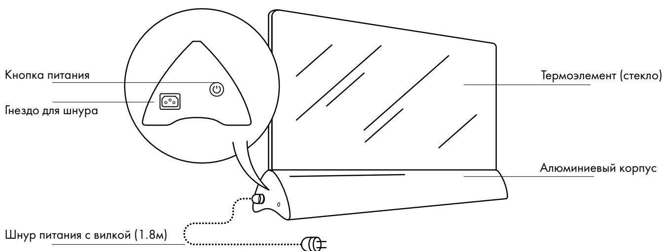
Рисунок 1. Обогреватель ThermoUp Floor/LED Plus
